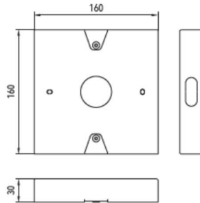
Aufputzadapter surface mounted adapter
