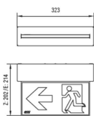
Deckenaufbau (DA) ceiling mounting (DA)
