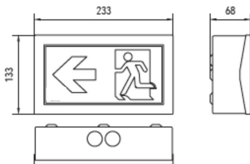
Wandaufbau (WA) IP40 wall mounting (WA) IP40
