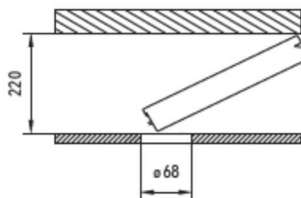
Deckenausschnitt und Einbautiefe section for ceiling flush mounting ceiling flush mounting depth
