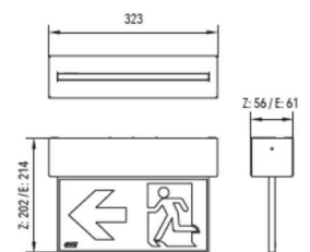
Deckenaufbau (DA) ceiling mounting (DA)
