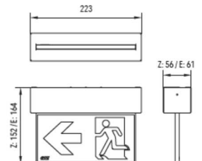
Ausschnitt für Deckeneinbau section for ceiling installation
