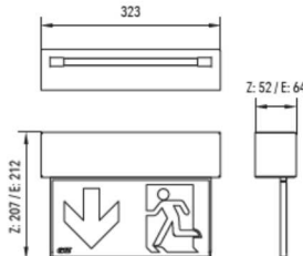
Wandaufbau (WA) wall mounting (WA)
